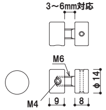
(六角レンチ・対辺2mm)
