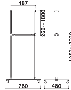
プリンタS30-A1との組み合わせ例
