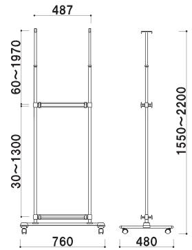
プリンバS30-A1との組み合わせ例
