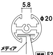
補修部品 F20用補強テープ 補強テープ材質 ■低発泡塩ビ F20用: 幅13mm × 厚み1mm 補修部品 4X-X004
