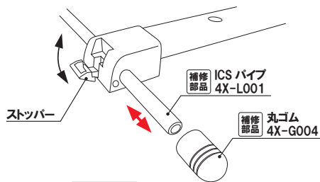
脚部構造図
