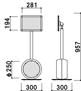
上部面板サイズ ■ W297 × H210(A4 ヨコ)
