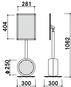
上部面板サイズ ■ W297 × H420(A3 タテ)
