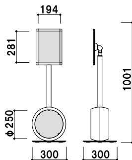
上部面板サイズ ■ W210 × H297(A4 タテ)
