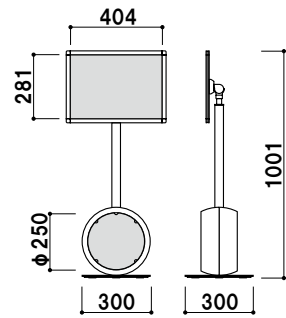
上部面板サイズ ■ W420 × H297(A3 ヨコ)
