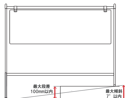
B-931 正面
