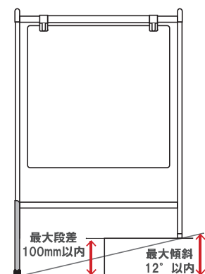
B-445・450 正面
